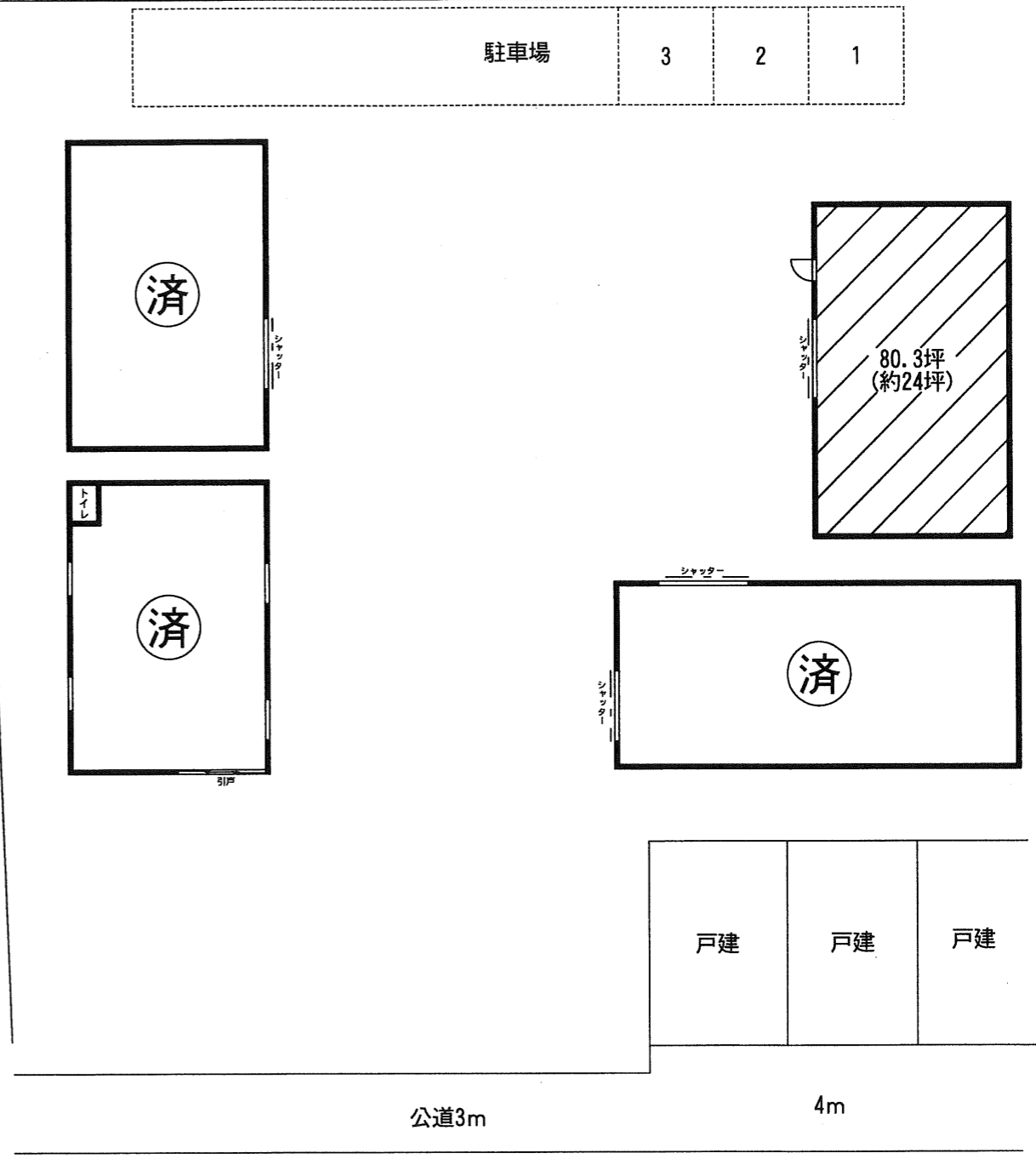
【配置図】
