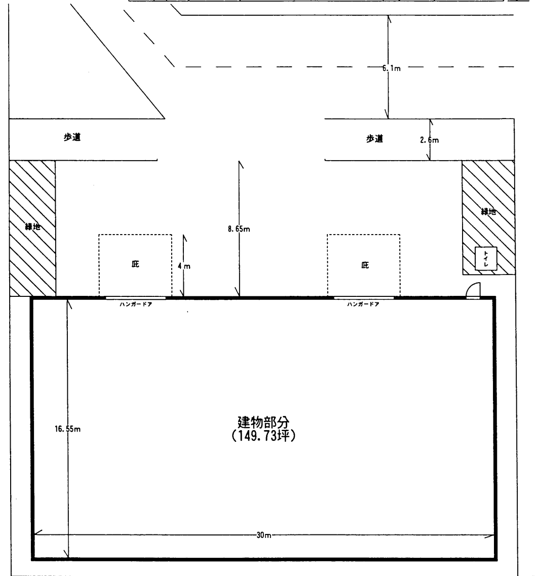
平面図
